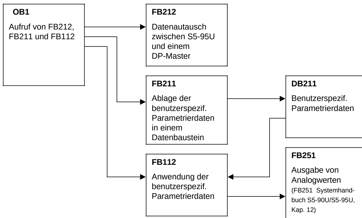
Bild 6.1 Programmstruktur
